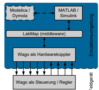
Abb. 1: Prototypischer Hardware-in-the-Loop Aufbau
